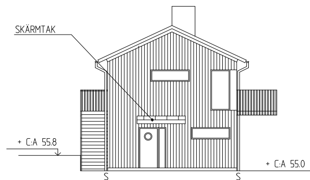
FASAD MOT SYDVÄST
