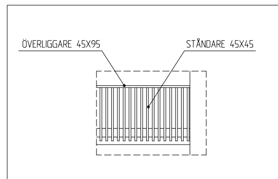
DETALJ A, RÄCKE
