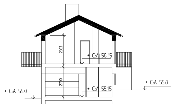
SEKTION A-A
