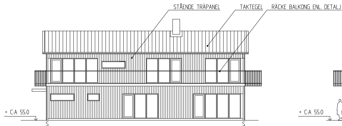
FASAD MOT SYDOST
