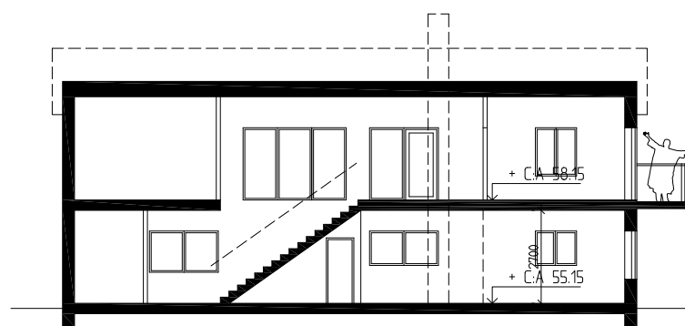
SEKTION B-B
